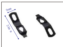
产品编号: PW20 产品名称: 小弹片
