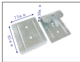
产品编号: J857530 产品名称: 镜框挂钩
