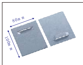
产品编号: J80100 产品名称: 镜挂
