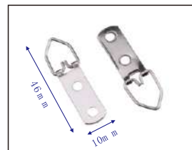
产品编号: E613 产品名称: 两孔小吊挂
