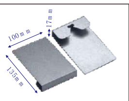
产品编号: J10017 产品名称: 镜挂
