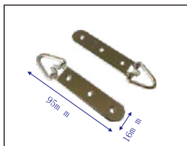
产品编号: E169528 产品名称: 三孔吊挂
